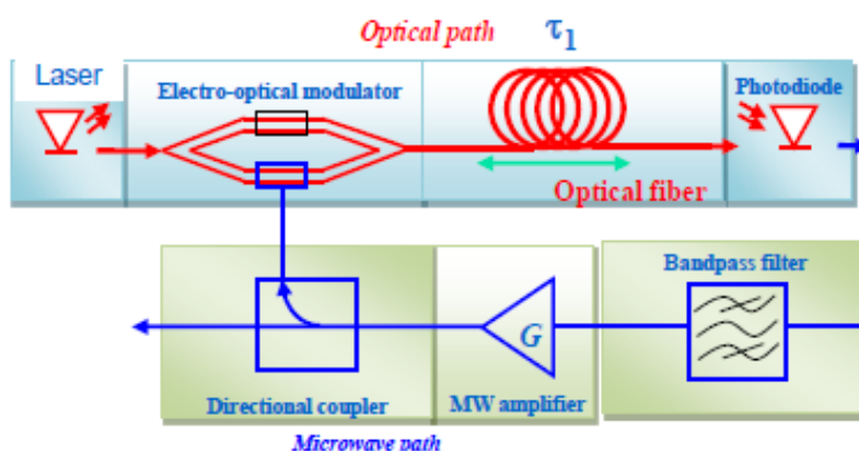
Рис. 1. Блок-схема радиофотонного СВЧ генератора.
