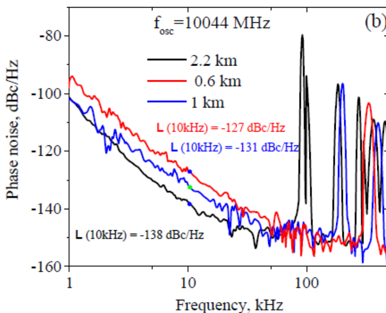
Рис. 2. Фазовые шумы спин-волнового оптоэлектронного генератора СВЧ сигнала на 10 ГГц.
